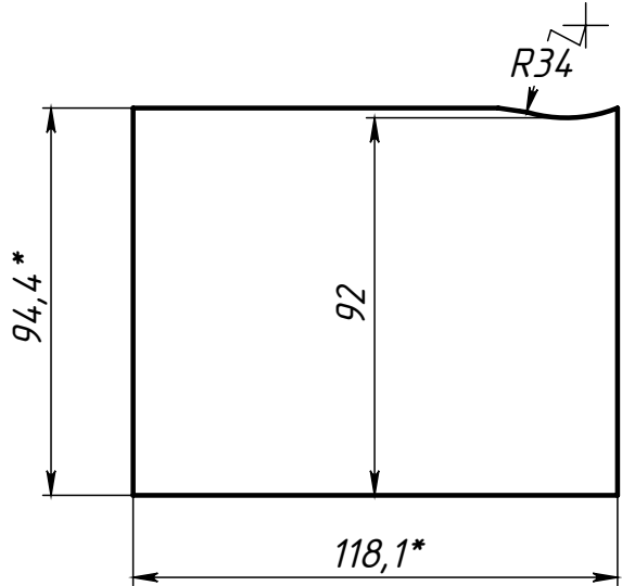
Поз.2 (Угольник)
